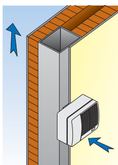
2 - KÖZPONTI CSŐVEZÉS
