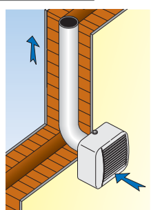
EGYÉNI CSÖVEZÉS
