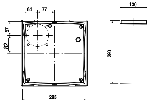
Beépítő-kit (rendelésre) 2SV0110
